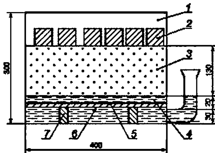
Г — сосуд; 2 — образцы; 3 — капиллярно-утолщенный песок; 4 — вода; 5 — гидравлический затвор; 6 — металлическая сетка; 7 — подставка
